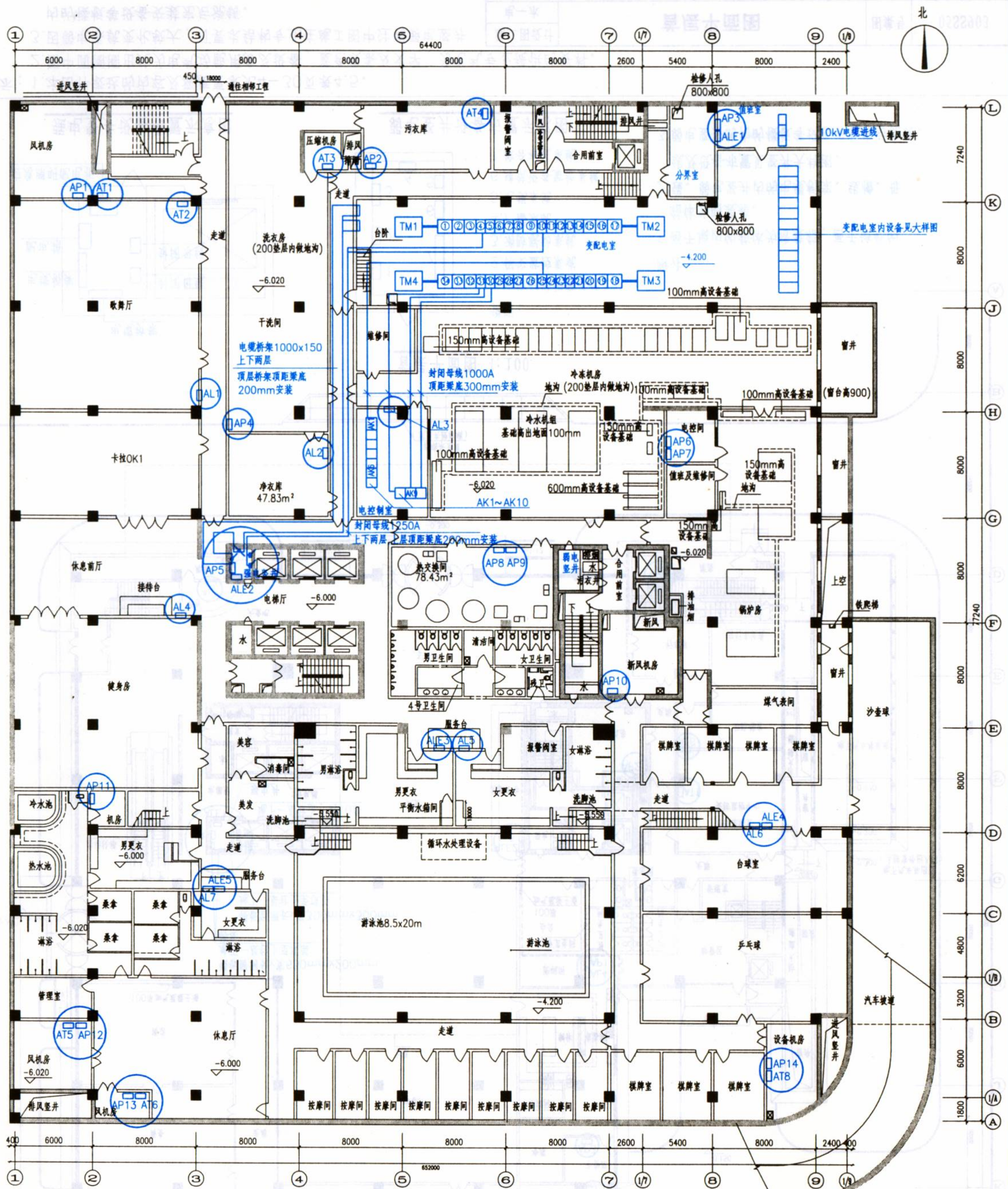
地下一层平面图 1:100
