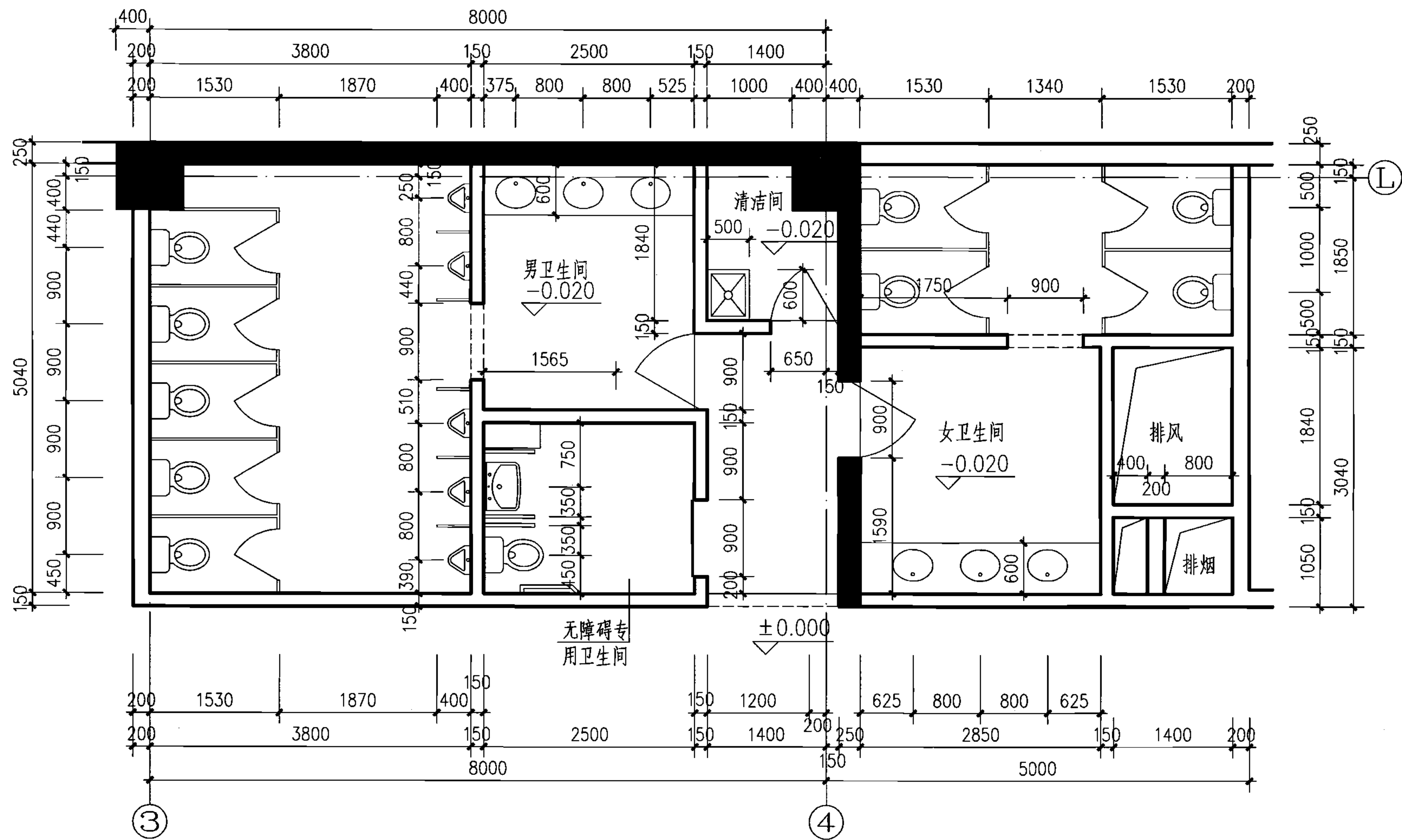
1号卫生间首层平面图 1:50
