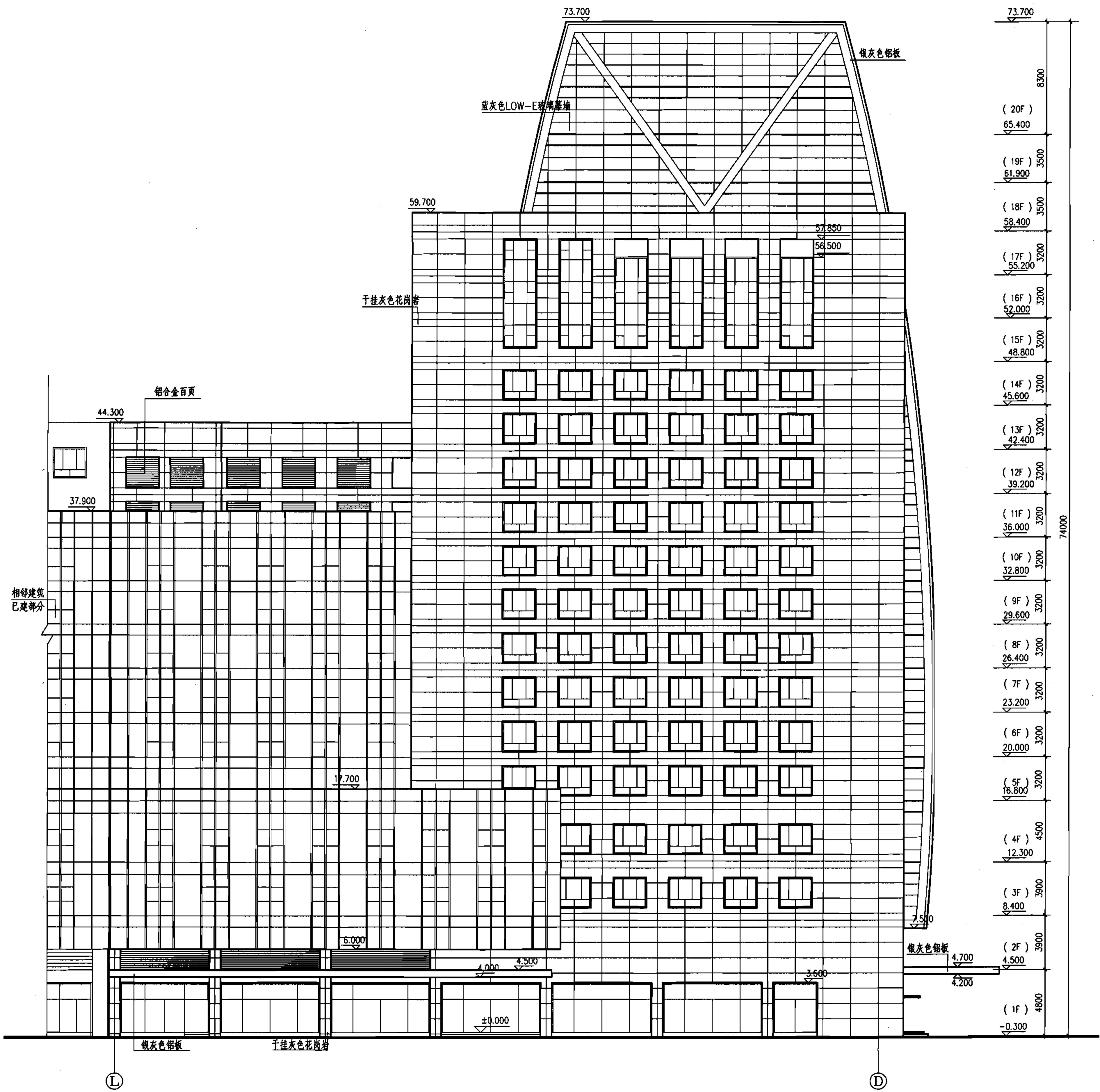
①-① 轴立面图 1:100
