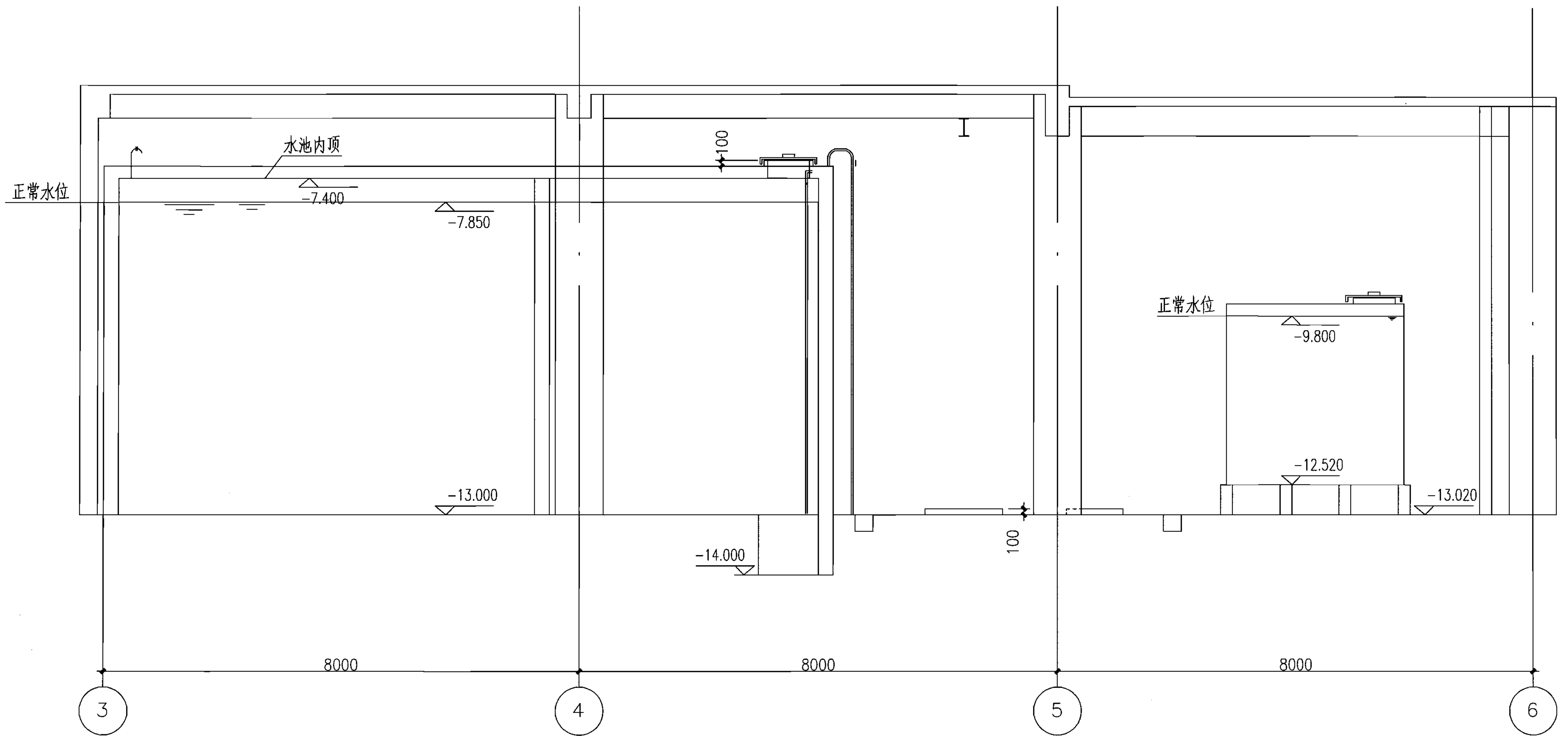
泵房、水池剖面图1-1 1:100
