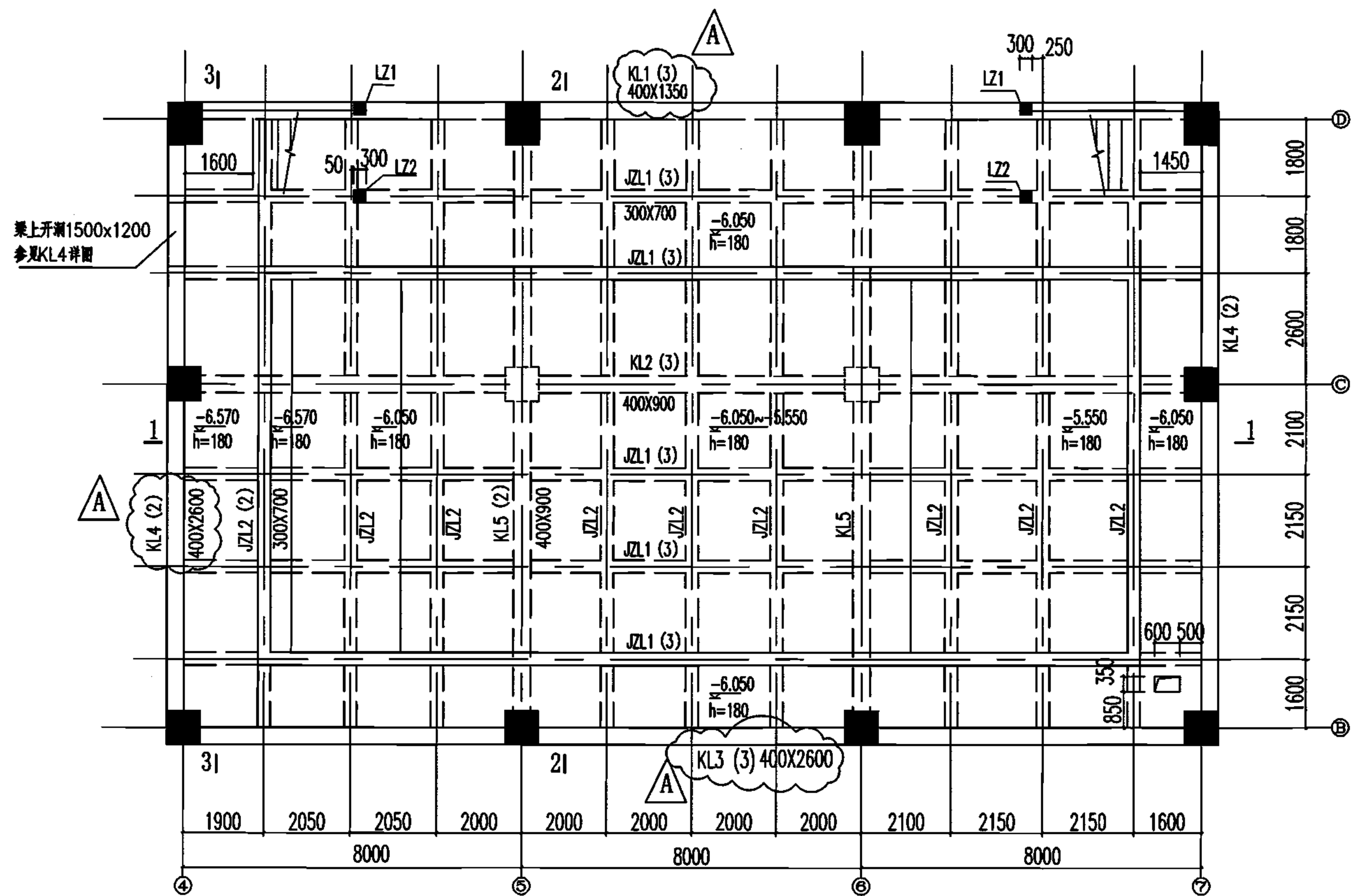
游泳池池底结构平面布置
