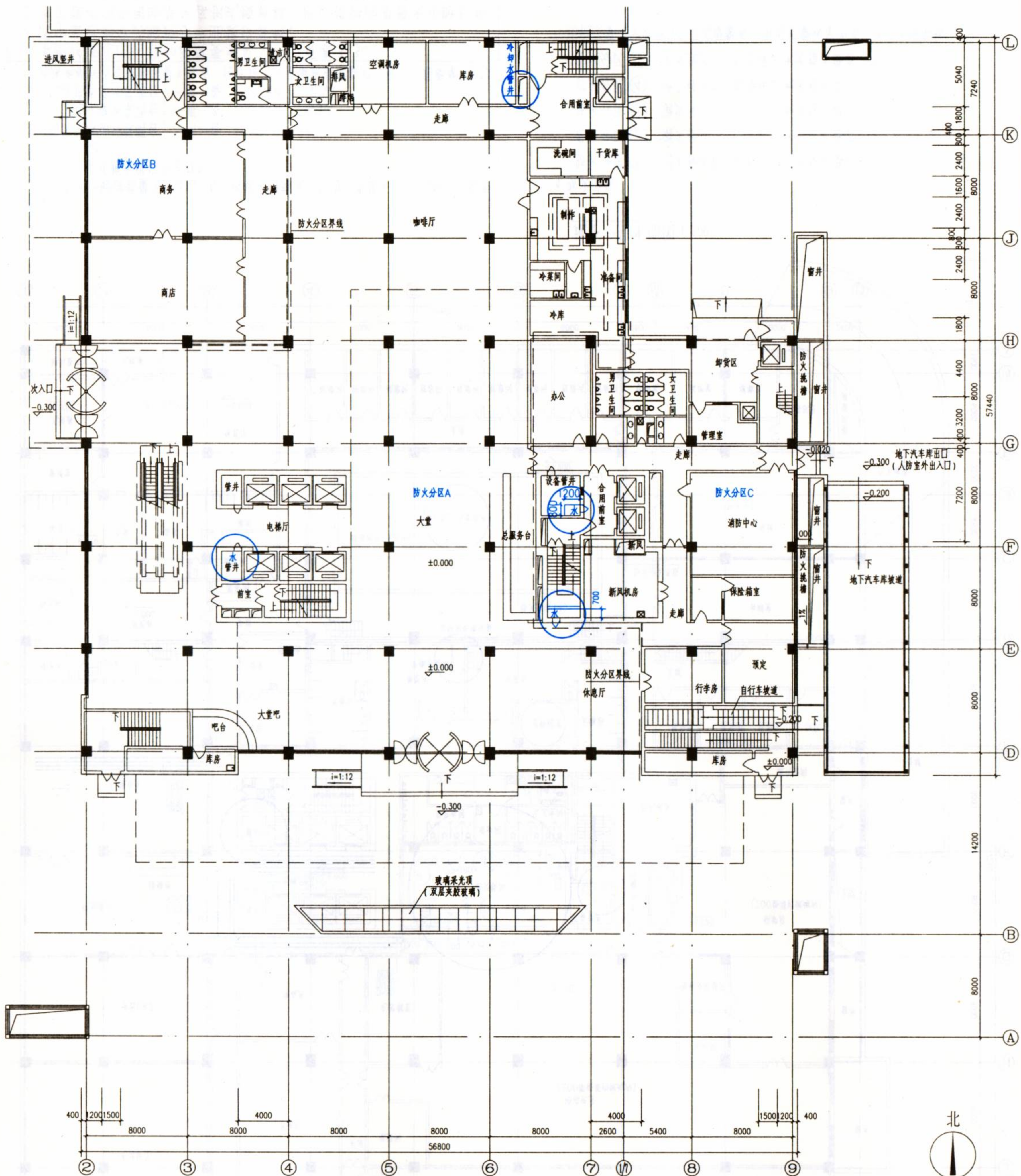
首层平面图 1:100
