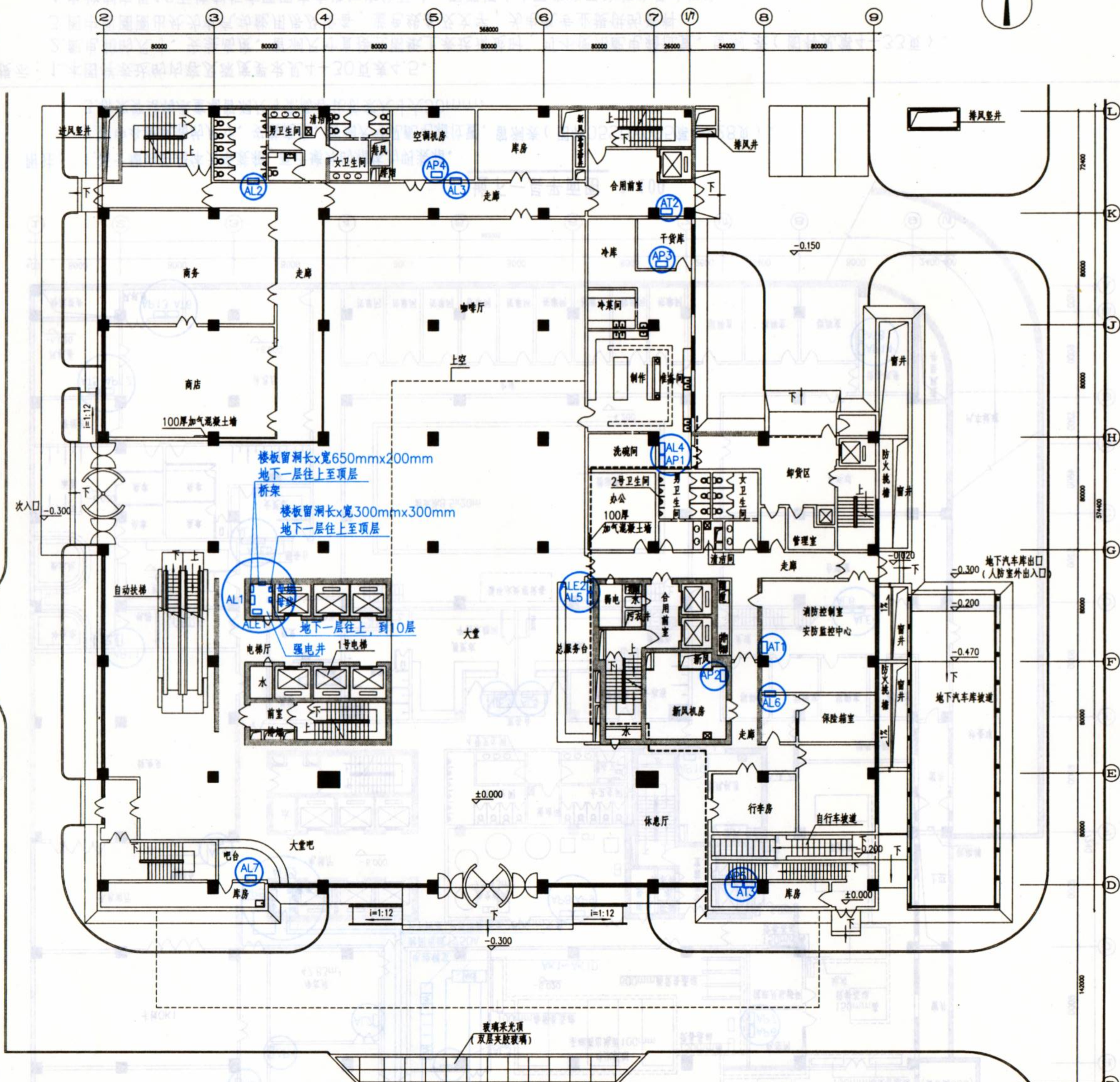
首层平面图 1:100
