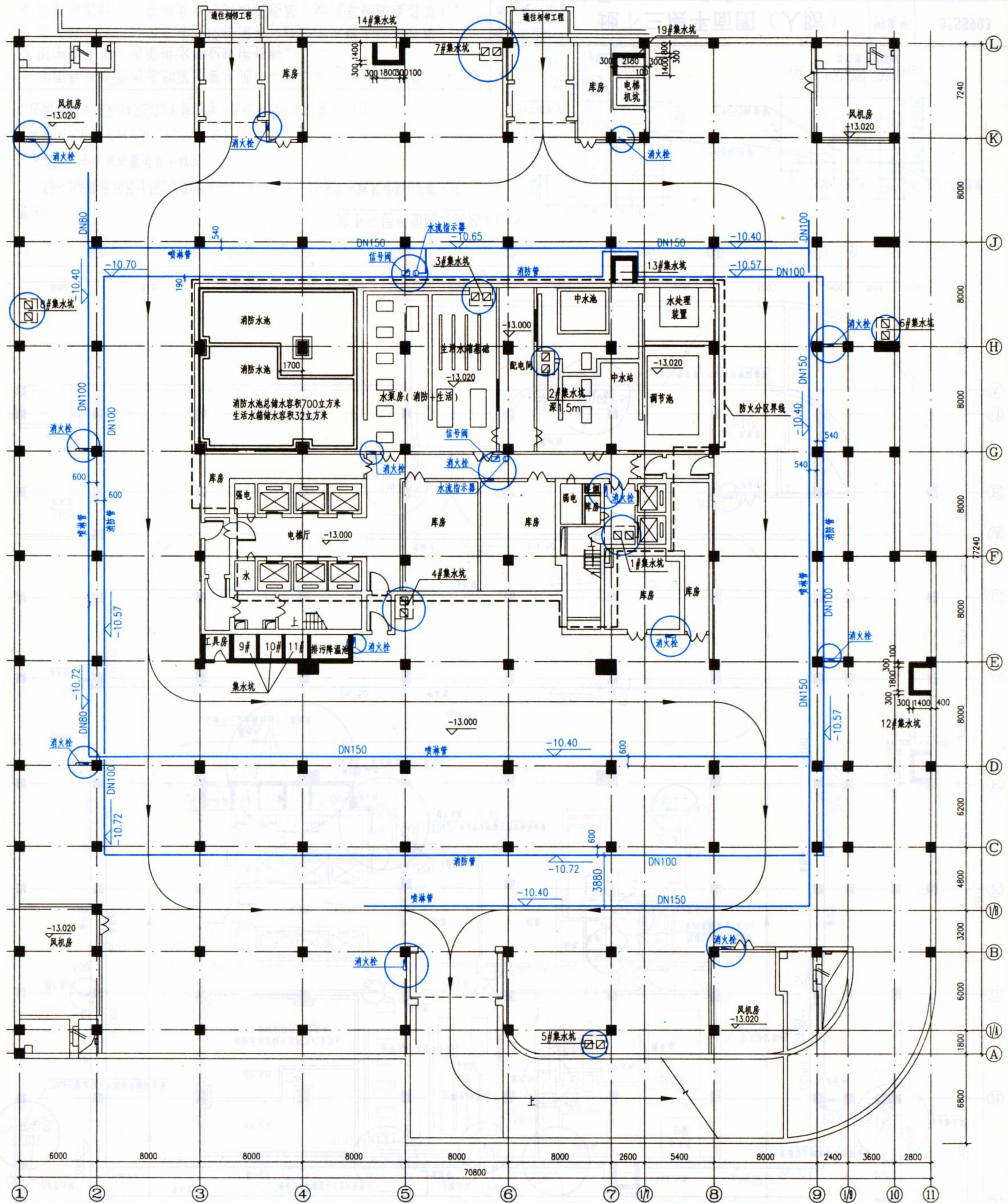
地下三层平面图 (人防) 1:100
