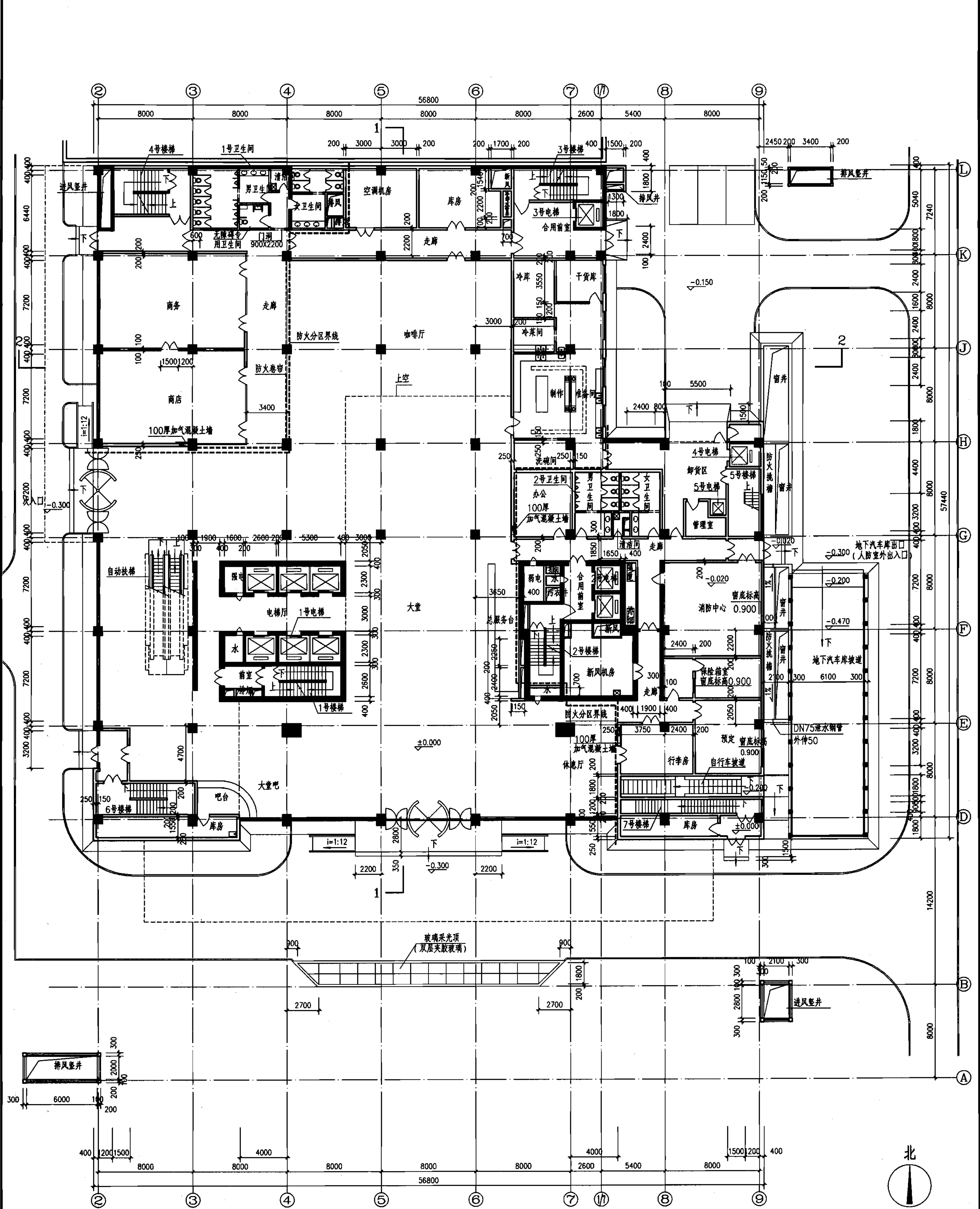
首层平面图 1:100 本层建筑面积: 2860m 2
