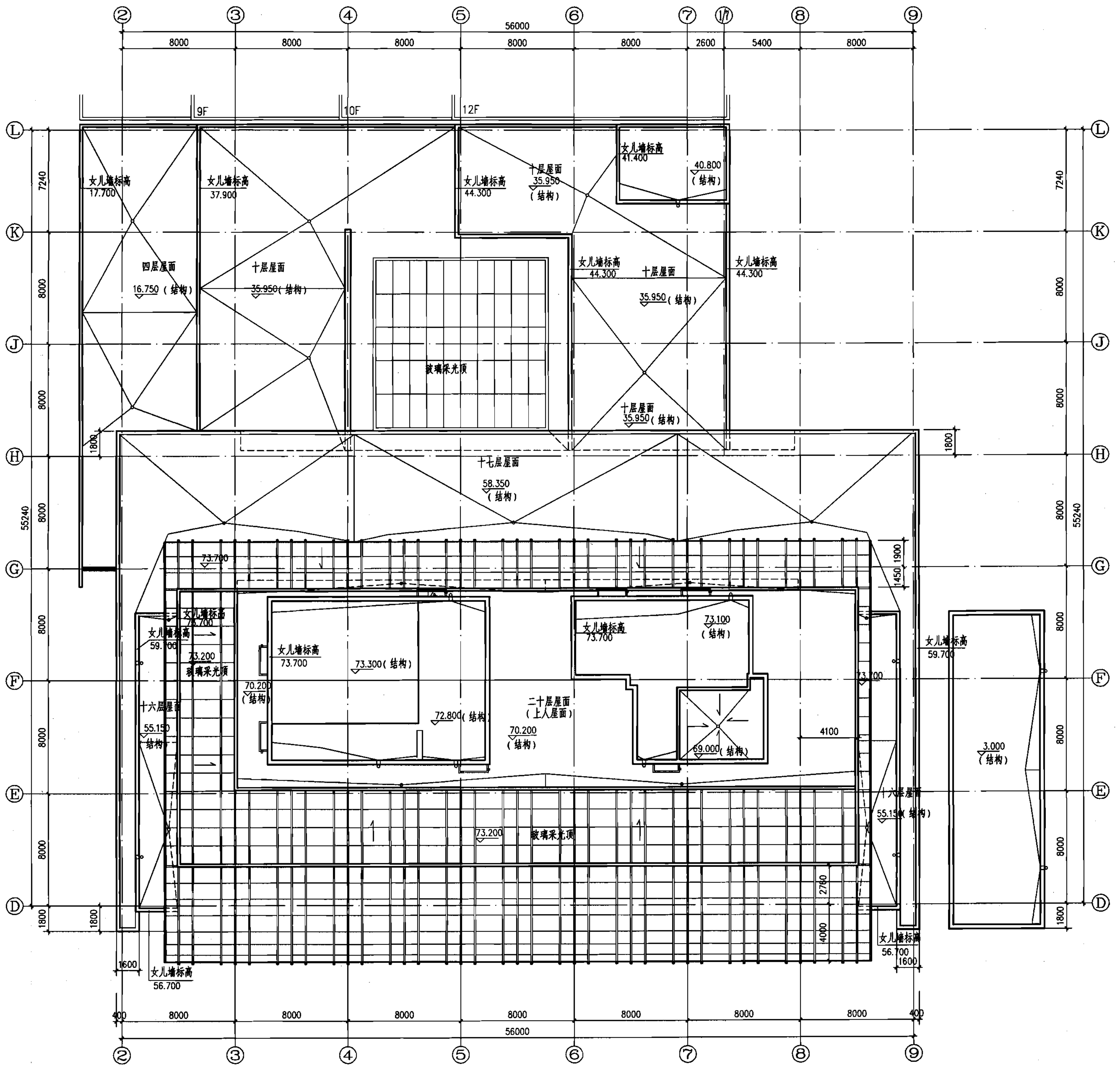
屋顶平面图 1:100
