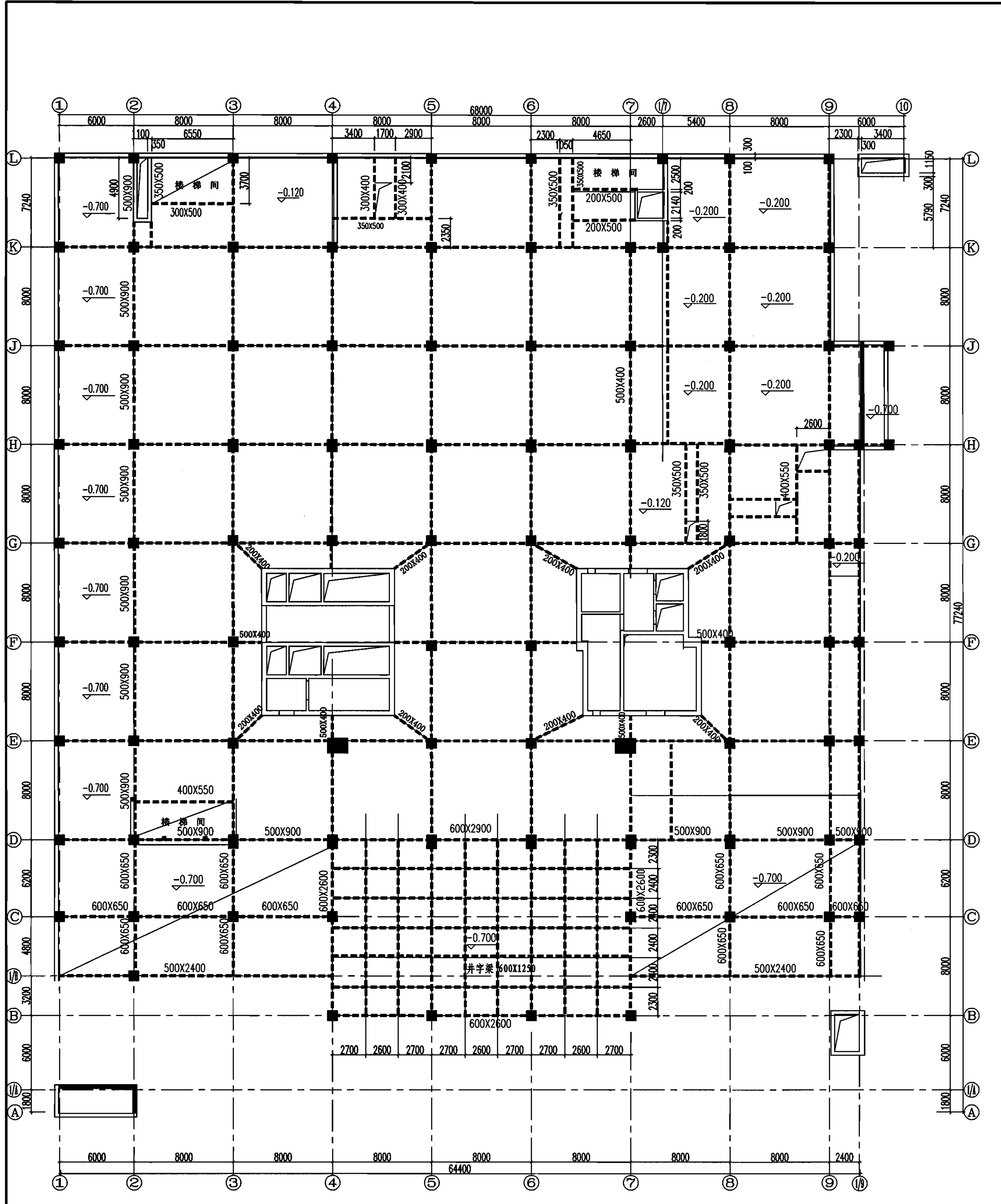
首层结构平面图
