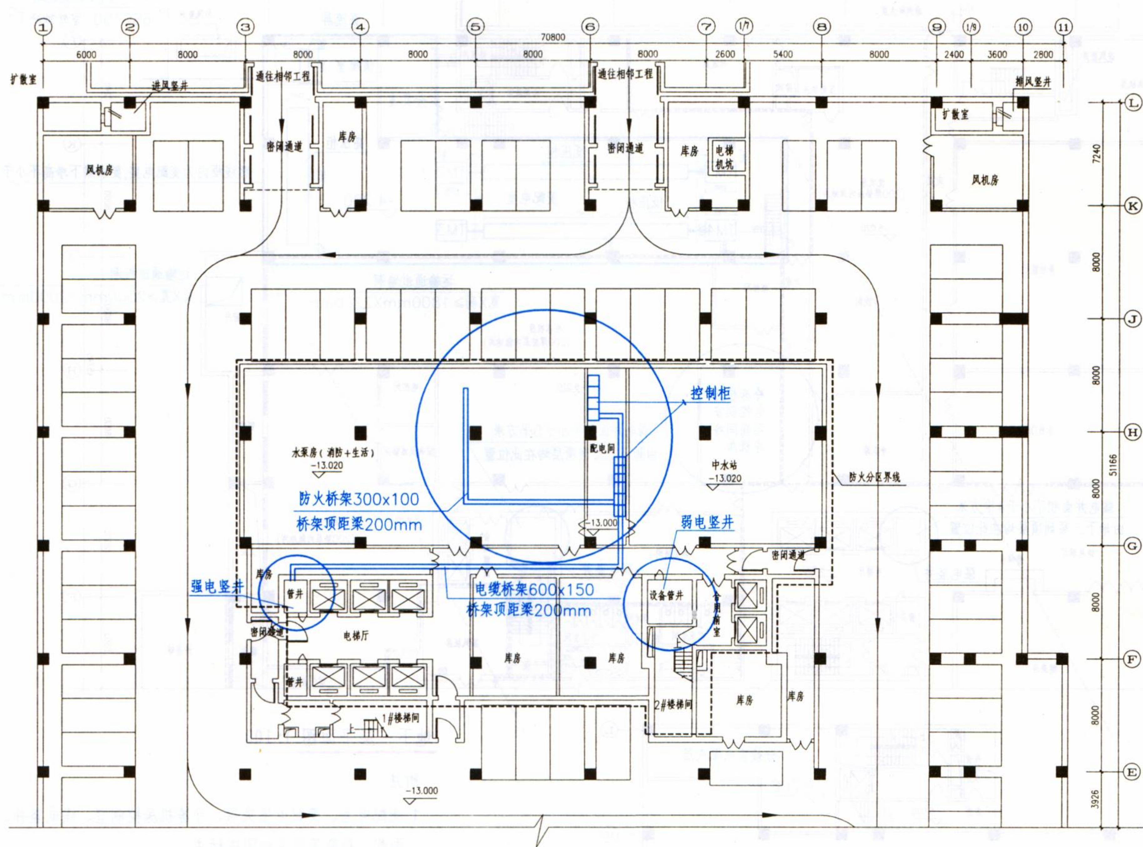
地下三层平面图 (人防) 1:100
