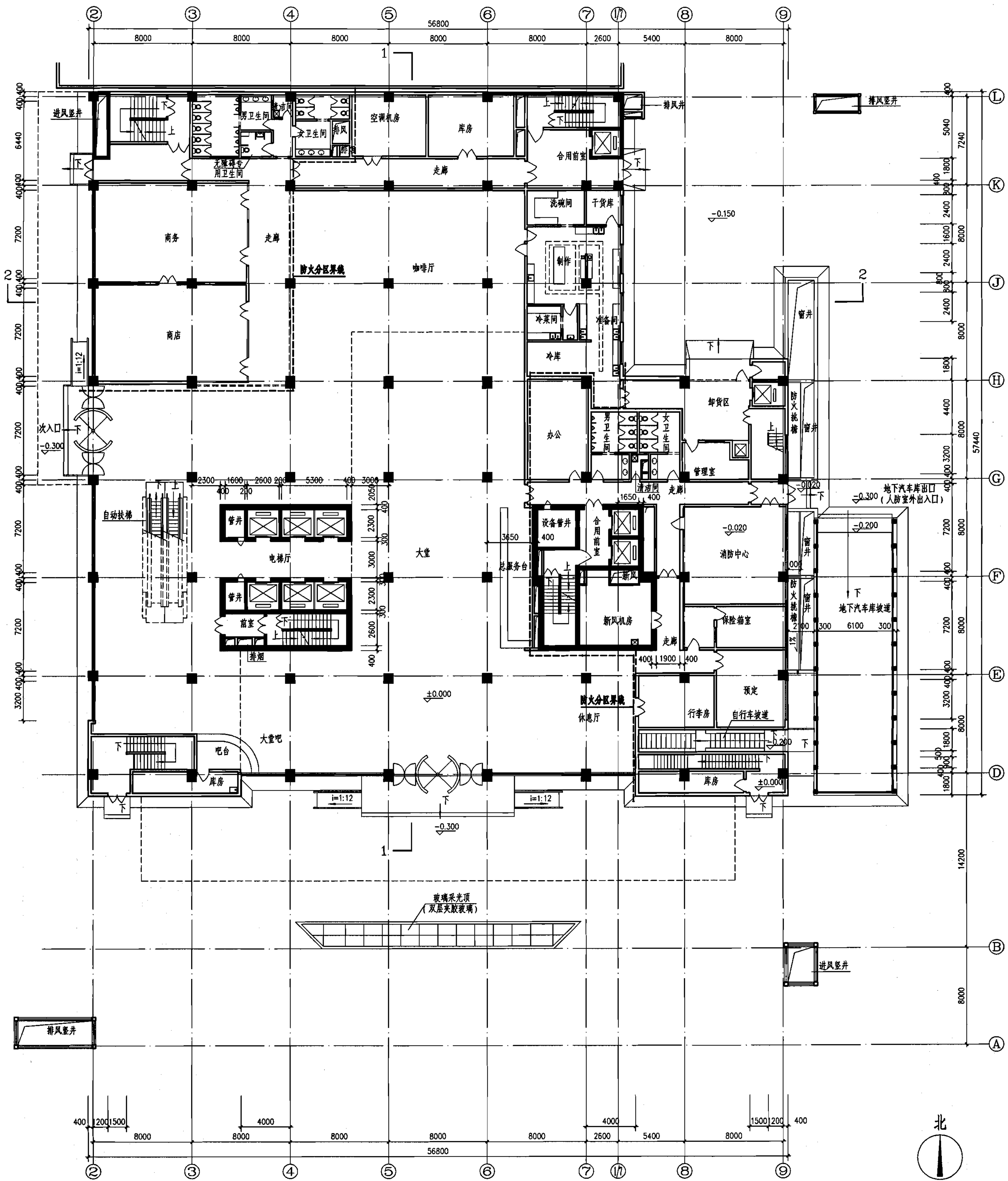
首层平面图 1:100 本层建筑面积: 2860m 2
