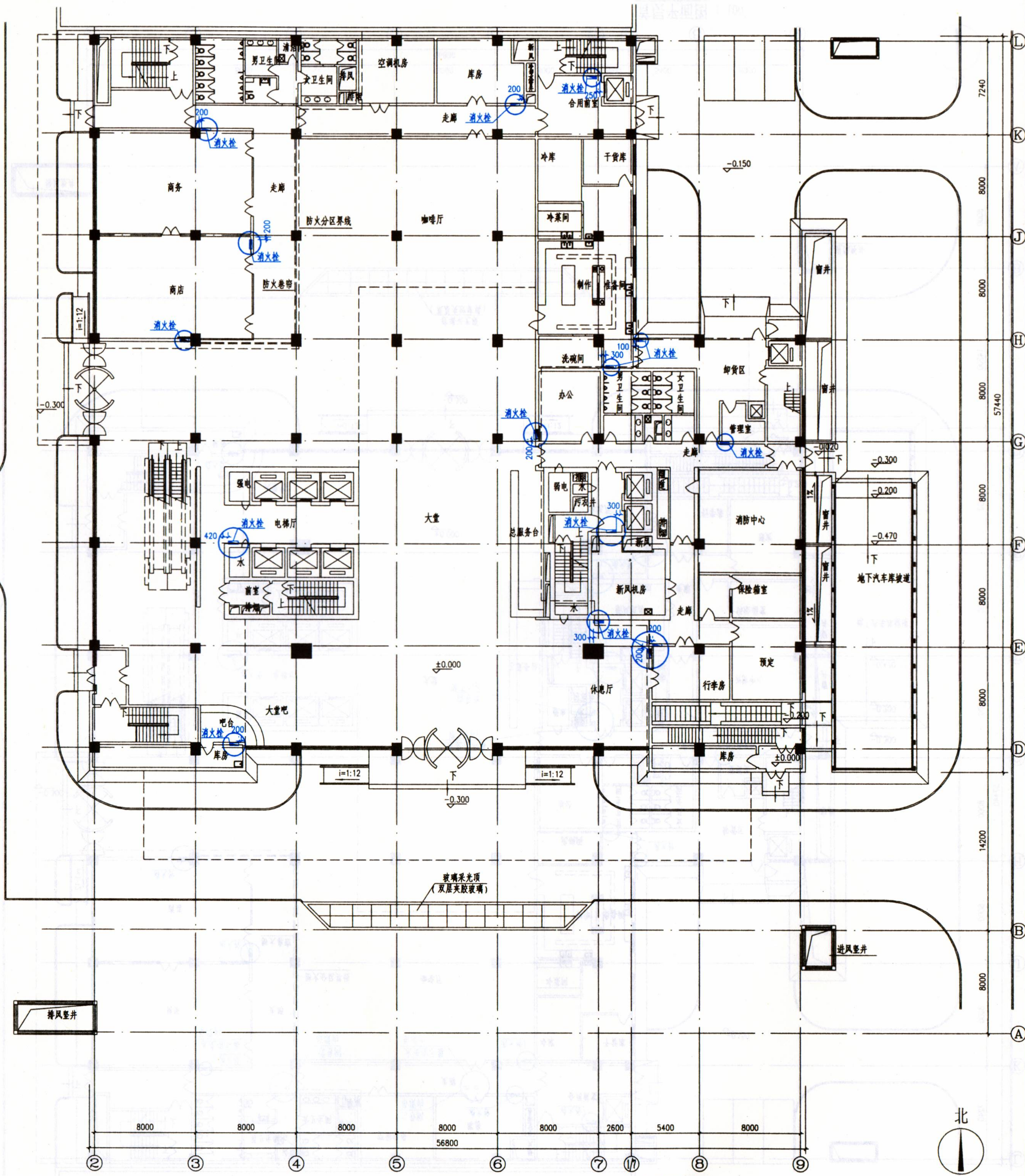
首层平面图 1:100 本层建筑面积: 2860m 2
