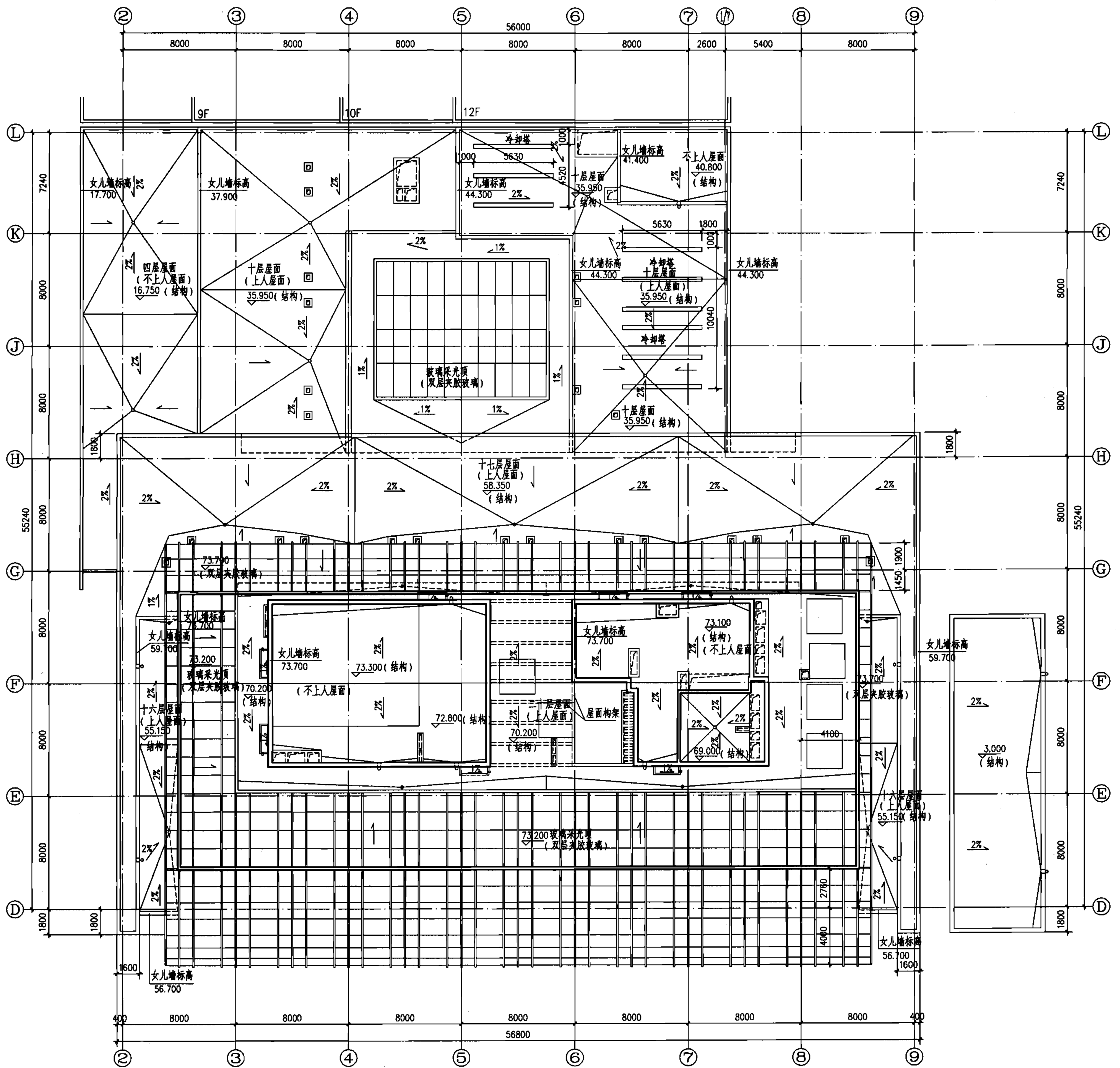
屋顶平面图 1:100
