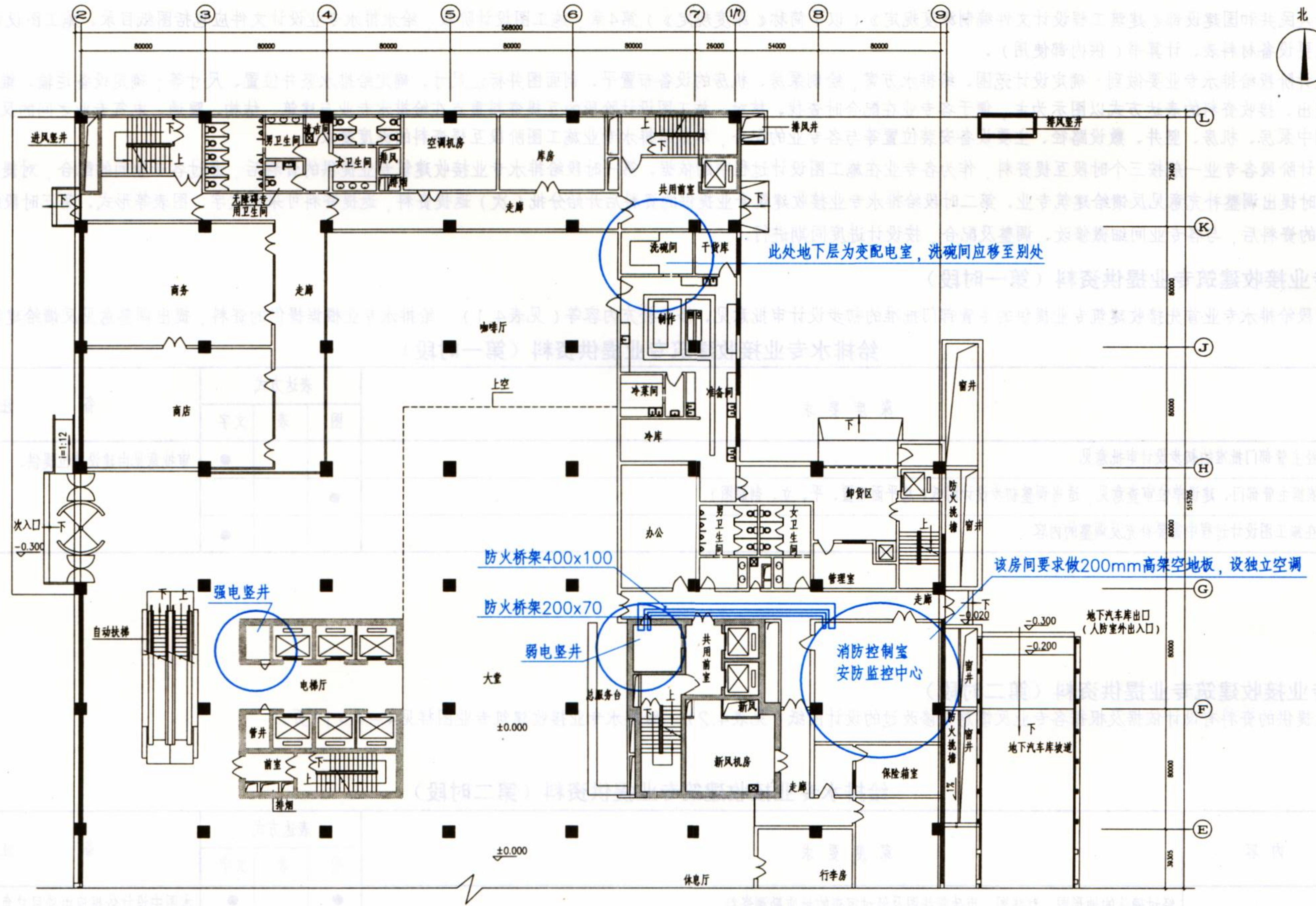
首层平面图 1:100
