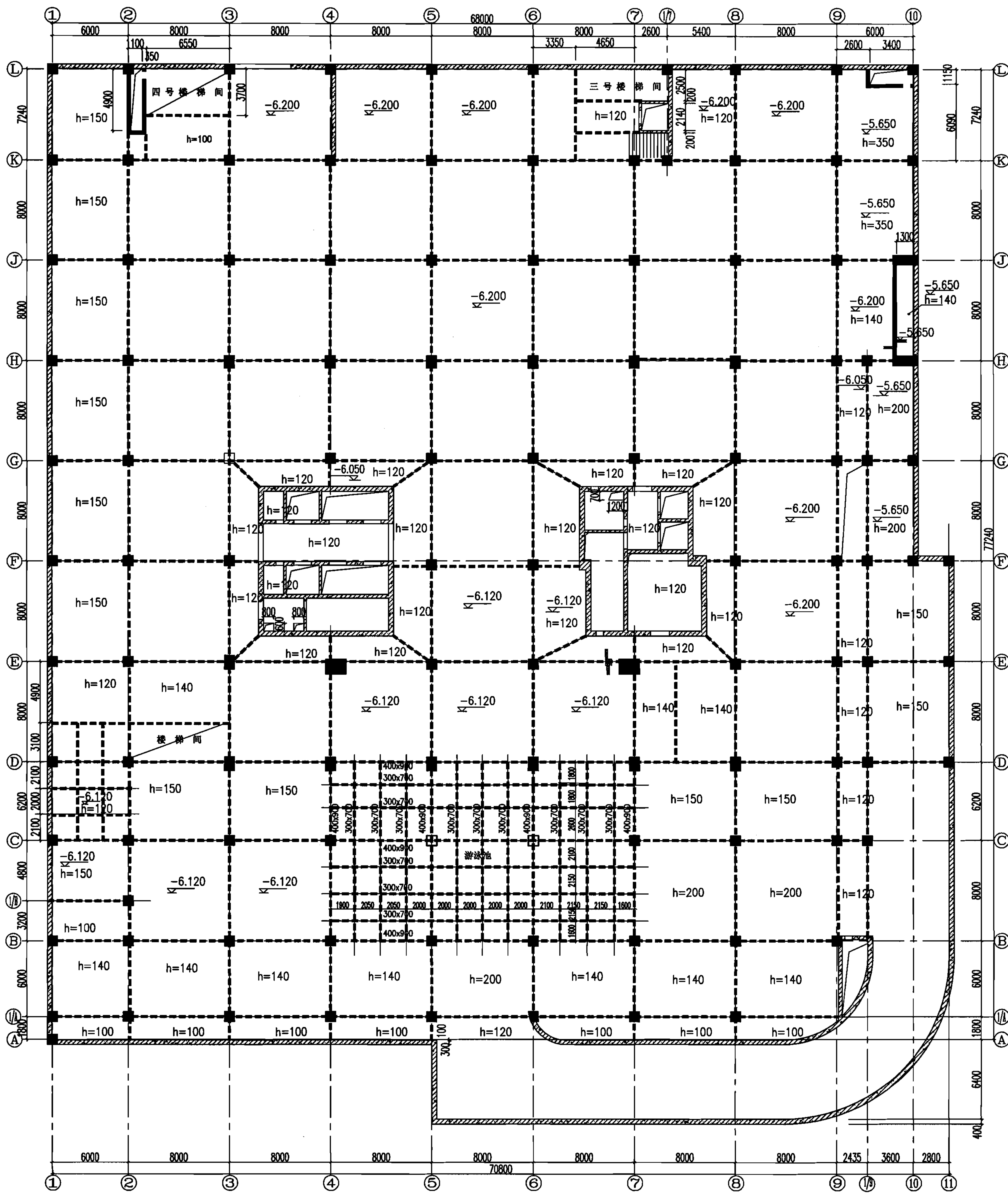
地下一层结构平面图 未注明结构标高为-6.050m
